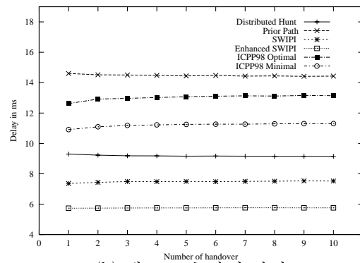
(b) 핸드오버 지연 시간
