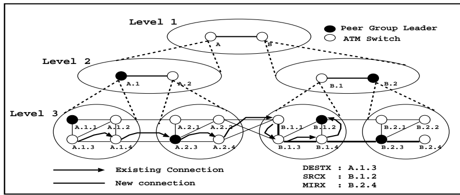
그림 2: PNNI 기반의 계층적 네트워크 구조와 라우팅의 예
