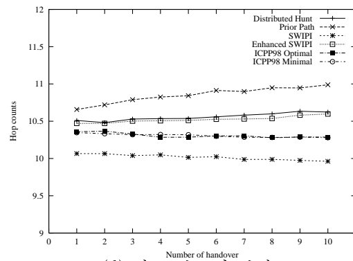
(d) 최종 경로의 길이
