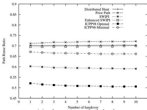
(c) 기존 경로 재사용 율
